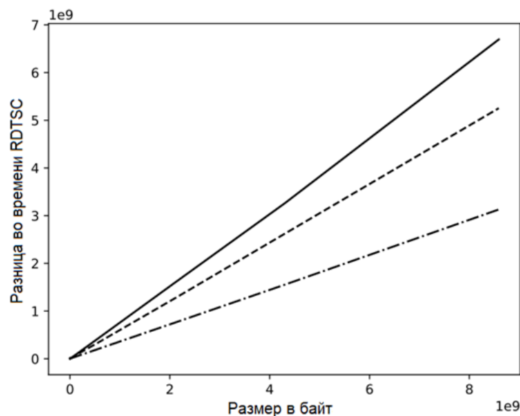
Рисунок 4 – Время, затраченное на выполнение сложения двух длинных величин с использованием параллельного алгоритма, показанного на рисунке 2, выполненного 36 логическими ядрами (пунктирная линия), сравнённое со временем, затраченным тем же алгоритмом, но таким, что каждый поток выполнял векторизованное сложение (рис. 3), создавая пару битов i и c для рекурсивного сложения с применением (4) (точка-пунктир), и со временем выполнения последовательного сложения с использованием инструкции ADC (сплошная линия)
