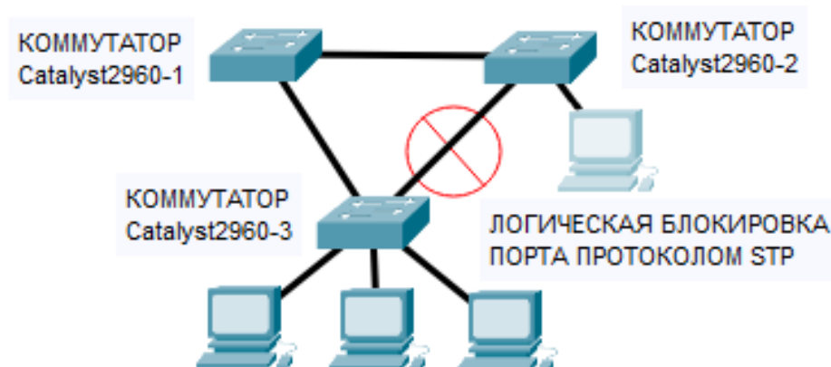
Рисунок 5 – Сегмент сети с резервным каналом без петли коммутации
