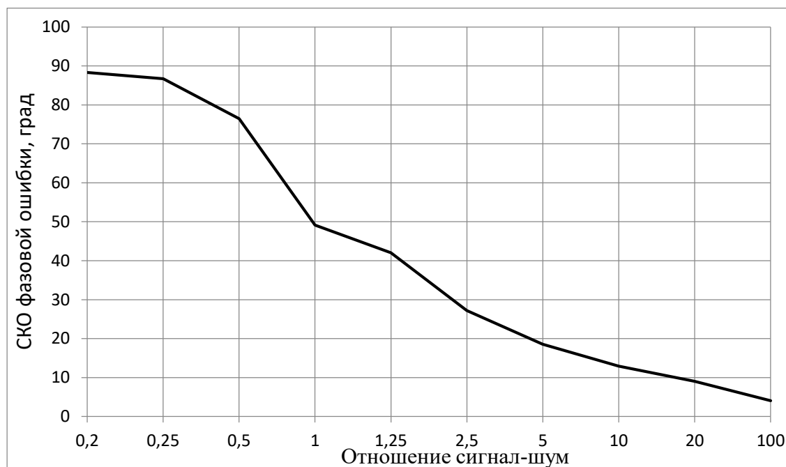
Рисунок 4 – Результаты расчёта влияния гармонической помехи со случайной фазой на СКО отклонения фазы при измерениях
