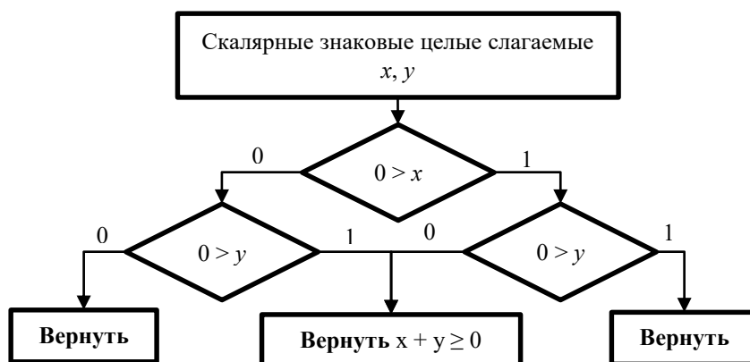
Рисунок 1 – Обнаружение флага переноса во время выполнения сложения целых со знаком в дополнении до двух
