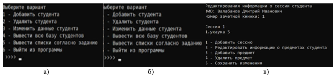
Рисунок 3 – Окна программы
