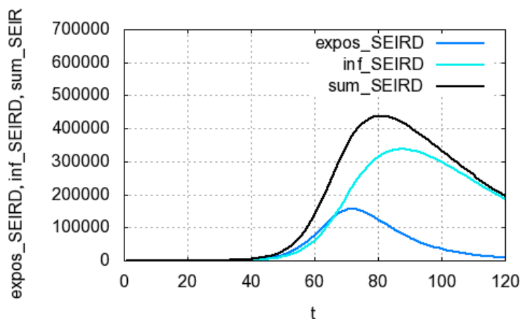
Рисунок 5 – Результаты расчета по SEIRD-модели
